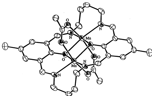
[Mn 2 (L 5 )(AcO) 2 ]
